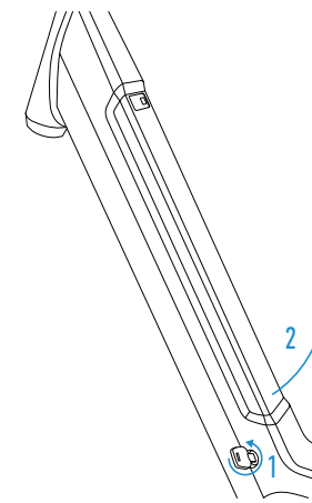
Bilde 13 - Fjerning av integrert batteri
