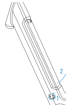
Рисунок 13 – Вытягивание интегрированной АКБ
