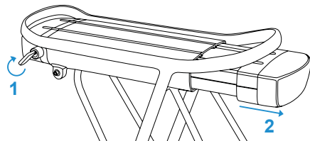
Obrazek 7 – Wyjęcie baterii bagażnikowej
